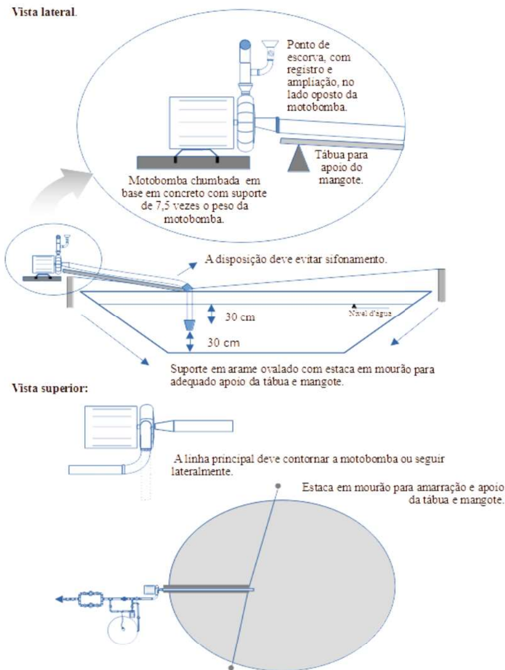
Figura D - Desenho esquemático da instalação do conjunto motobomba, com o cuidado necessário para a disposição do mangote de sucção em um reservatório e o esmero de não formar “barriga ou sifão” em sua disposição ao longo da linha de sucção. A ancoragem deve ser realizada preservando o comprimento do mangote e a melhor disposição para o aproveitamento do reservatório. A tubulação de recalque e escorva deve evitar ficar por cima do motor, de modo a evitar que supervenientes vazamentos possam promover curto circuito.
