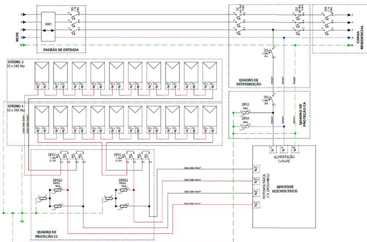
Figura O – Diagrama multifilar sugerido de sistema fotovoltaico do tipo “on-grid”.
