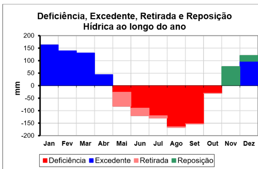
Figura 1 – Extrato do balanço hídrico climatológico para o município de Palmas (TO), município próximo a Tocantínia (TO), demonstrando os meses em que há excedente, retirada, reposição e déficit hídrico.
