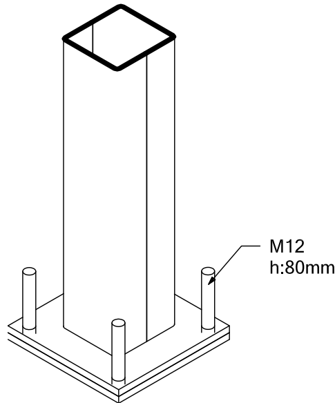
DET. A10045 Chapa Base macho M12 Compr. 80mm ESCALA
