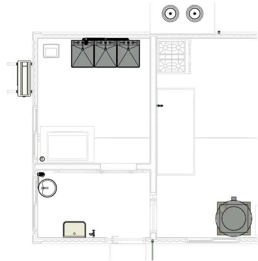
PLANTA PAV. TÉRREO - ÁGUA FRIA
