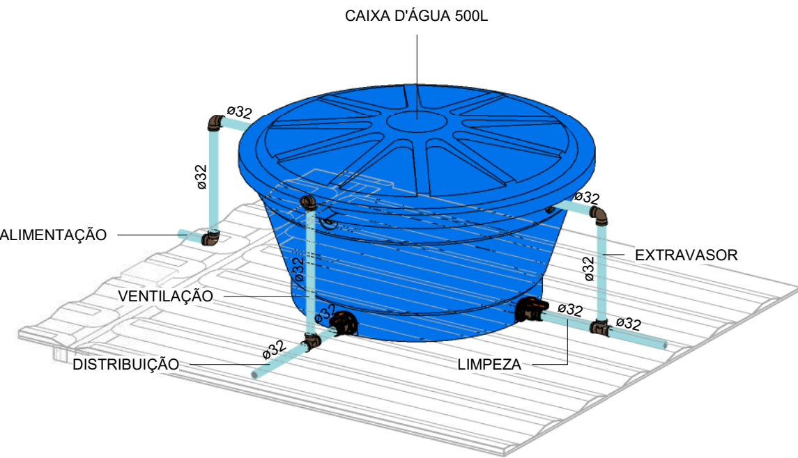
DETALHE RESERVATÓRIO
