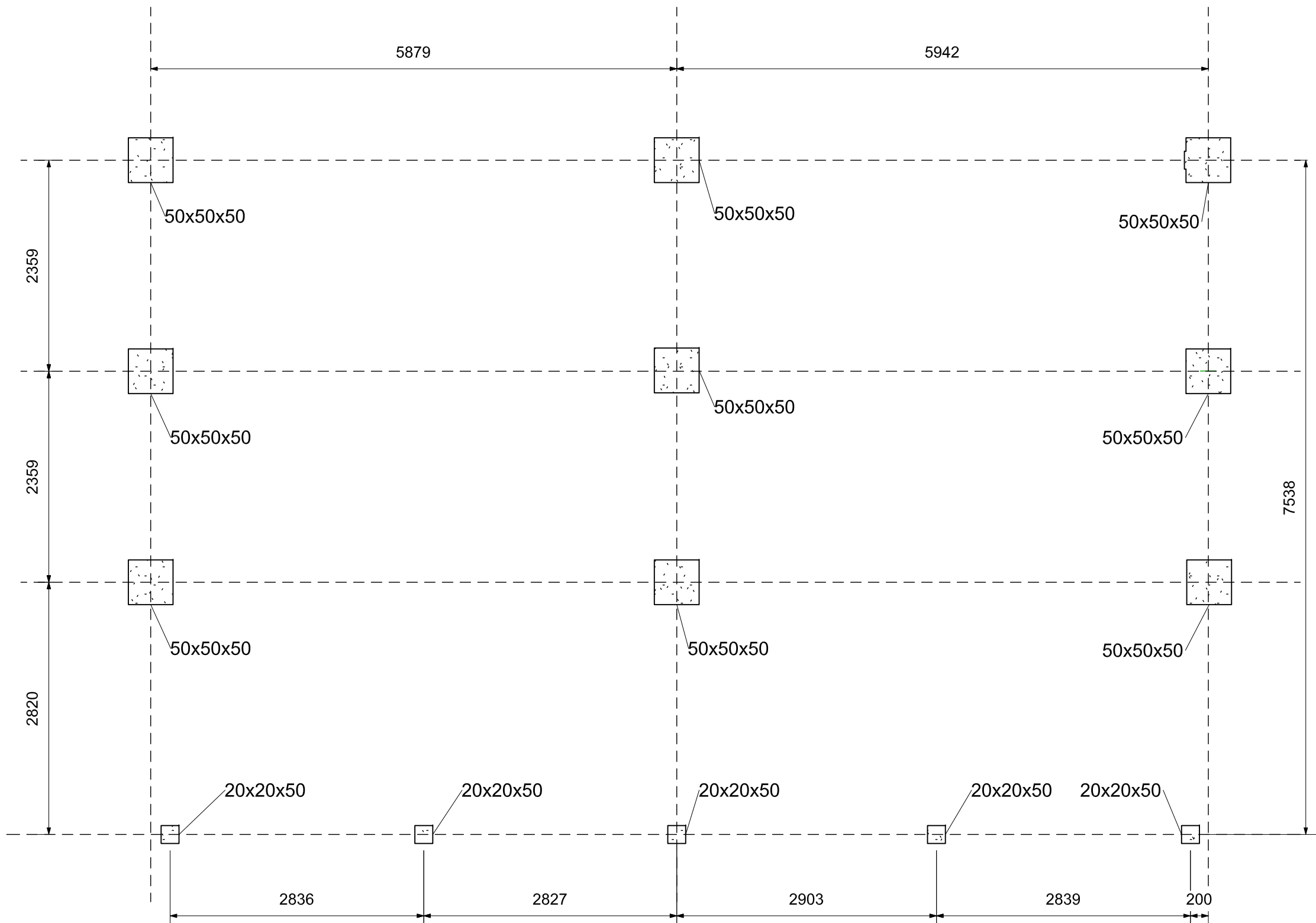
Bloco de Fundação em concreto armado 25 MPa, vergalhão 10mm CA-50 Fundação Container e Telhado ESCALA 1:50
