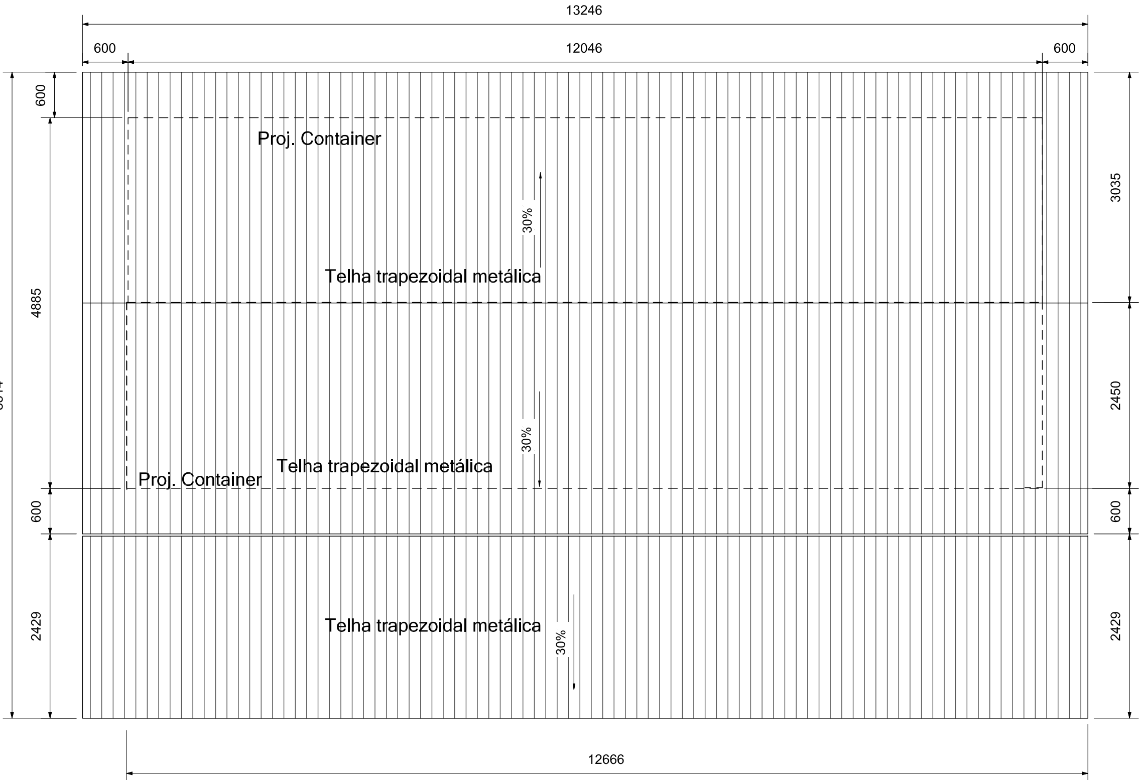
Planta de Cobertura ESCALA 1:50
