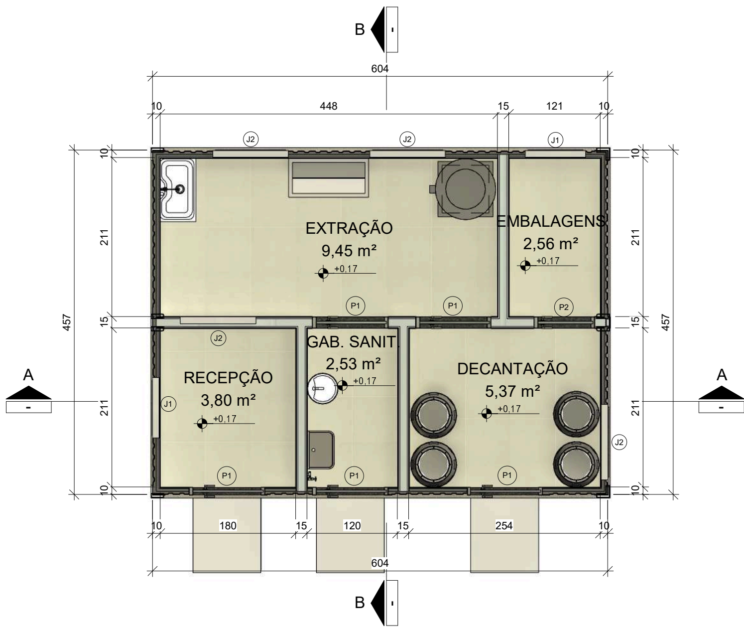
PLANTA PAV. TÉRREO
