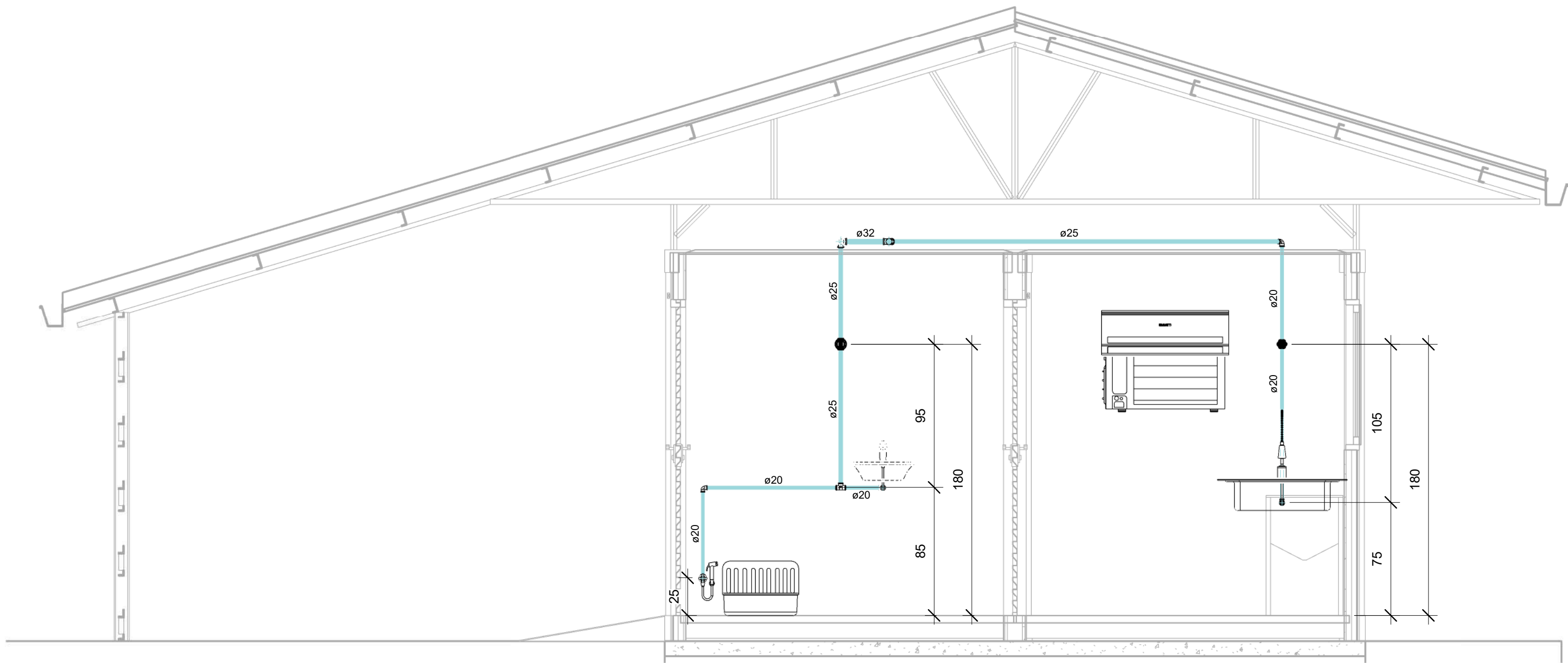
CORTE AA - ÁGUA FRIA
